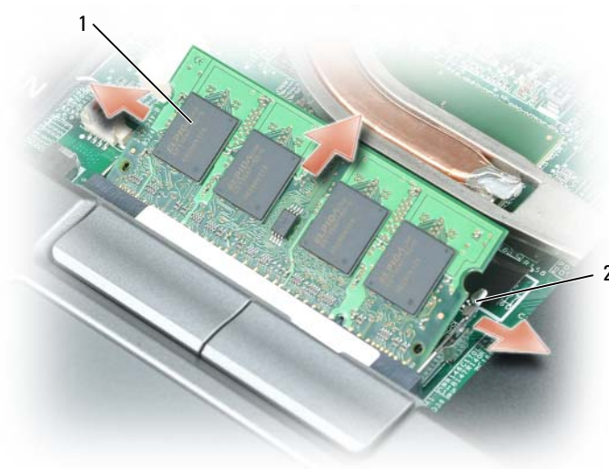
1 module de mémoire 2 clips de fixation (2)
