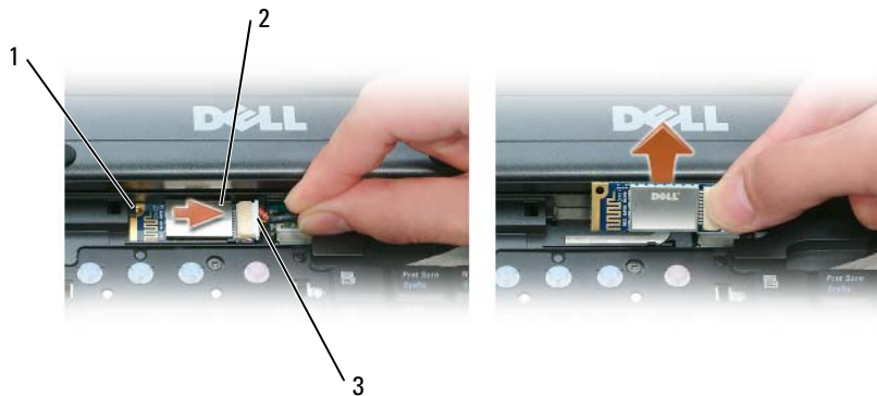
1 languette métallique 2 carte 3 connecteur de câble
