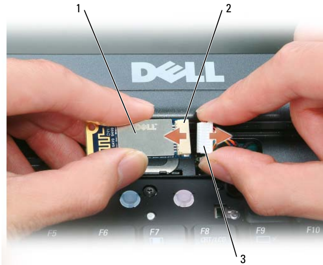
1 carte 2 connecteur de carte 3 connecteur de câble
